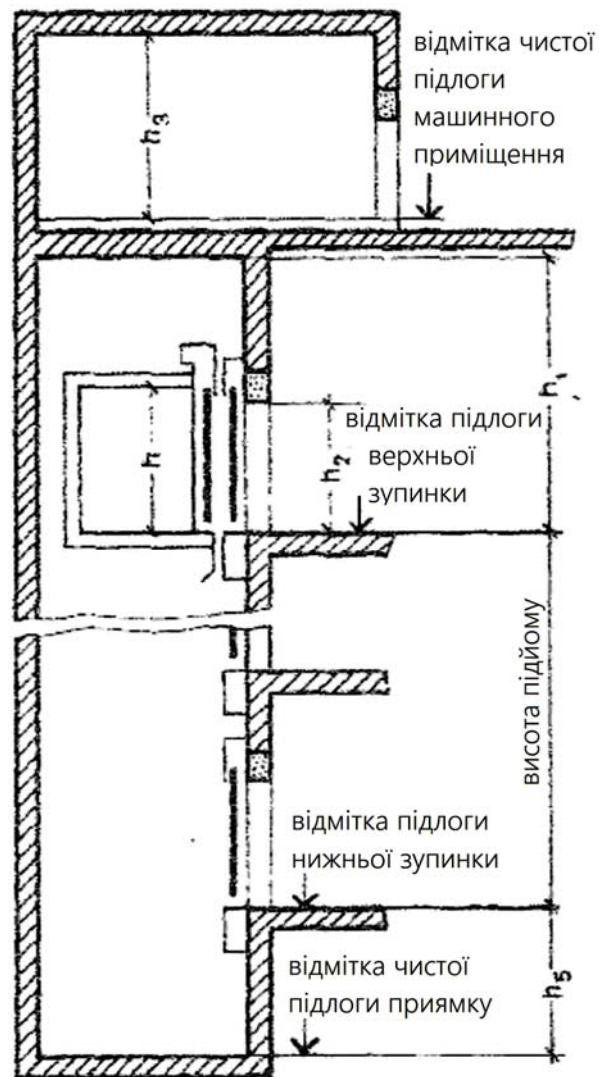
б) – розріз по шахті ліфту
