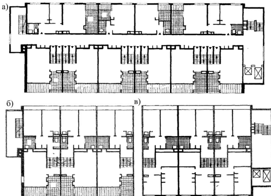
Рис. 6. Коридорний житловий будинок з перепадом рівнів в половину поверху: а) план коридорного поверху; б) план поверху над коридором; в) план поверху під коридором.
